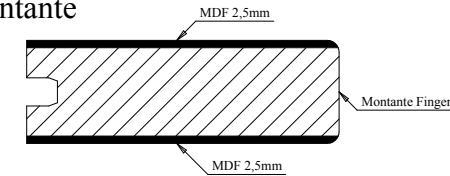
Montante
