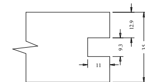
Moldura P-8mm
