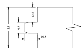
Respiga P-8mm
