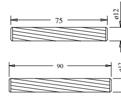
Cavilha
