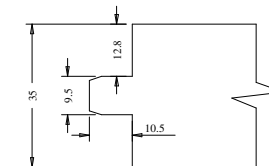
Respiga P-8mm
